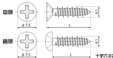
●サビに強いコンクリートビス
